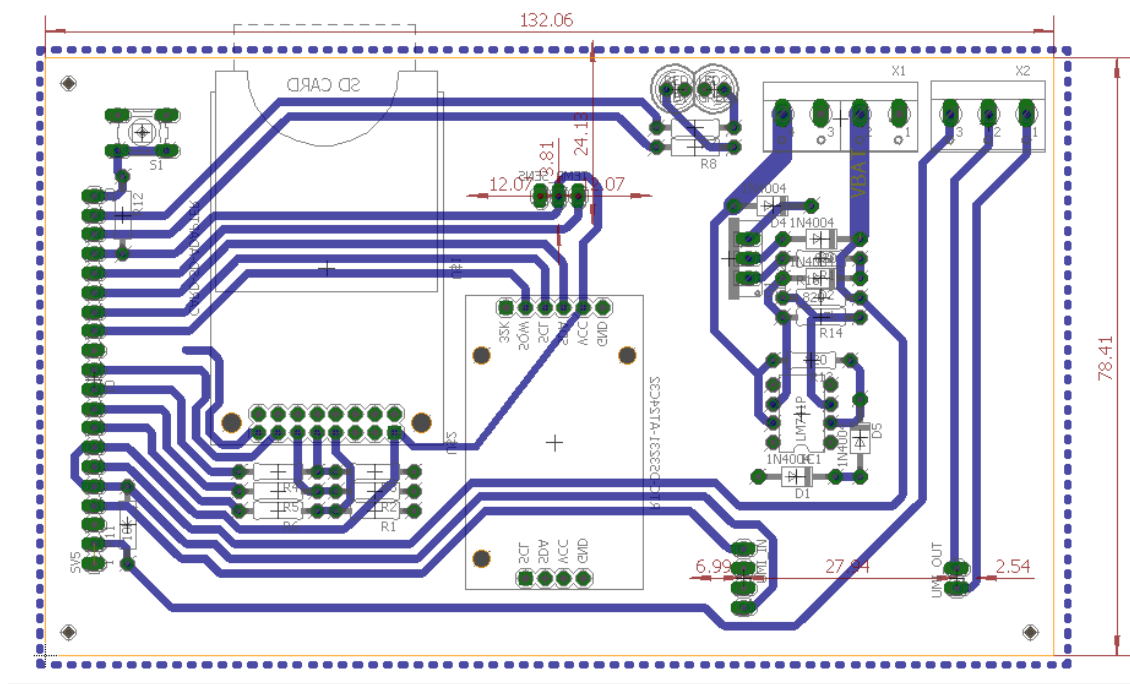
Figura 2: Design da PCI realizado no software Eagle.
